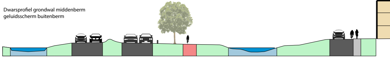
Dwarsprofiel geluidsscherm middenberm grondwal buitenberm
