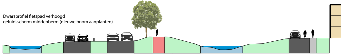
Dwarsprofiel hoog geluidsscherm buitenberm
