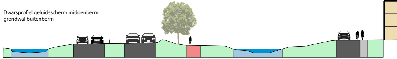
Dwarsprofiel fietspad verhoogd geluidsscherm middenberm (nieuwe boom aanplanten)
