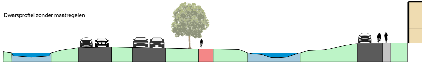
Dwarsprofiel grondwal middenberm geluidsscherm buitenberm
